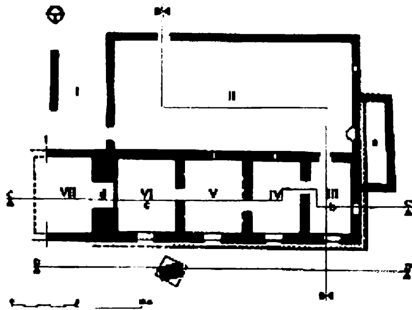
الشكل ٥ : مخطط حمام البارة من: G.CHARPENTIER, 1999
